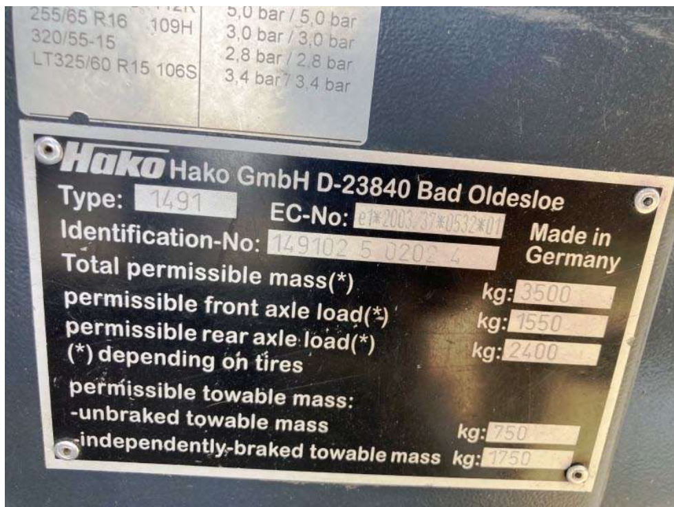
Bild 8 Typenschild
